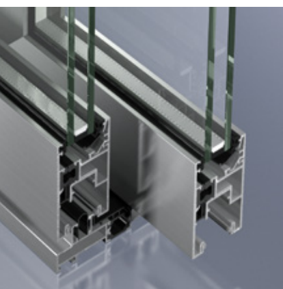
旭格ASS 50推拉系统 Schüco Sliding System ASS 50
