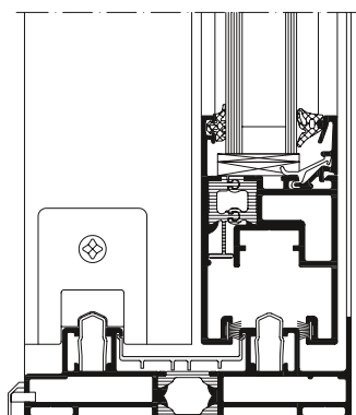
旭格ASS 50推拉系统 比例1:3 Schüco Sliding System ASS 50, scale 1:3
