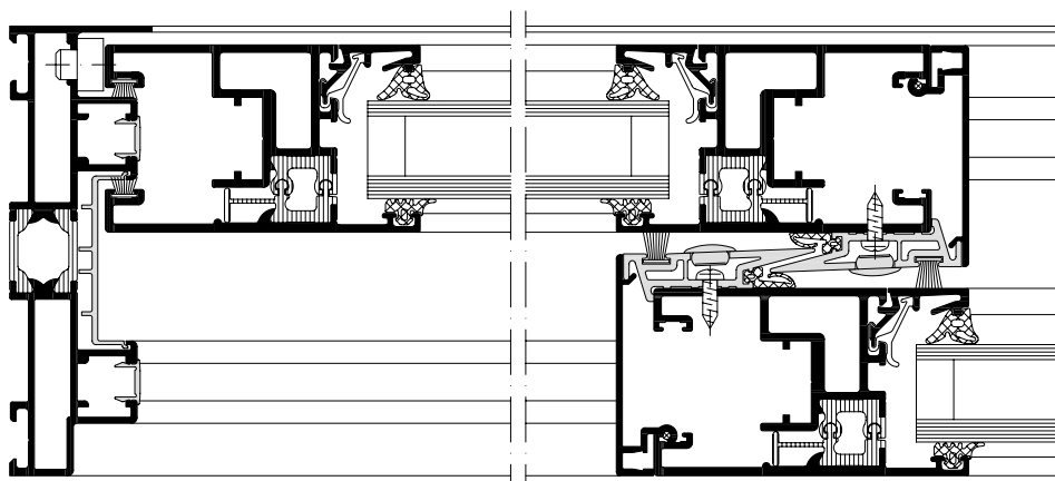
旭格ASS 50推拉系统，比例1:2 Schüco sliding system ASS 50, scale 1:2
