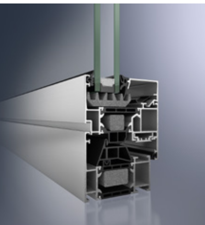
旭格AWS 70.HI窗系统 Schüco Window AWS 70.HI
