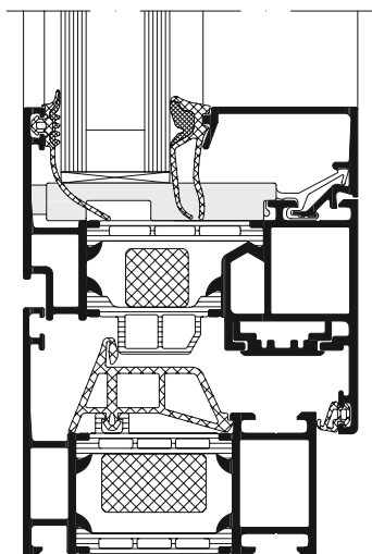
AWS 70，比例1:2 AWS 70, scale 1:2
